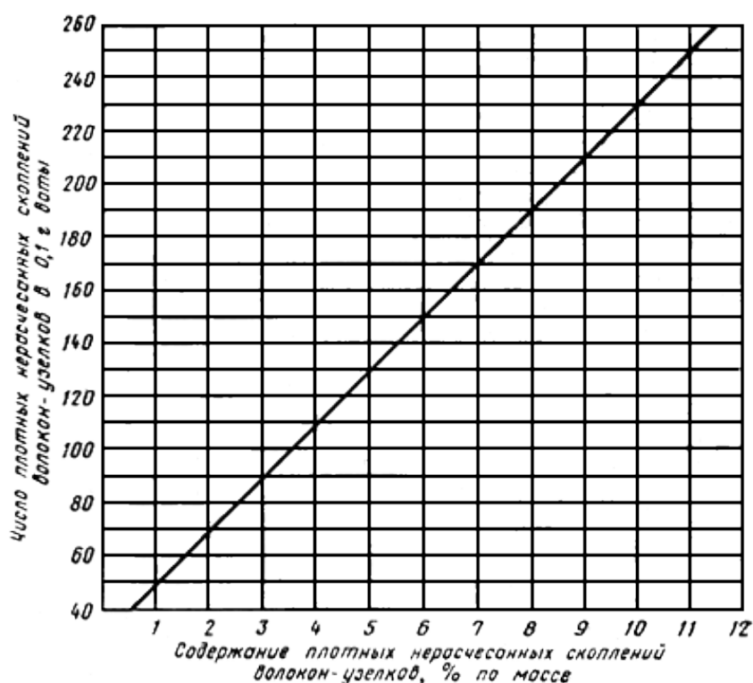
Рисунок 1 – Номограмма для определения содержания плотных нерасчесанных скоплений волокон-узелков в медицинской гигроскопической вате
