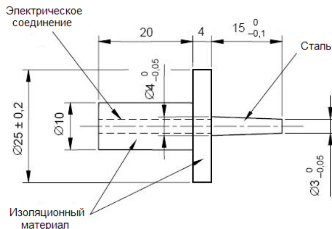
Рисунок 8 – Испытательный штырь (См. 8.4.2 d) )
