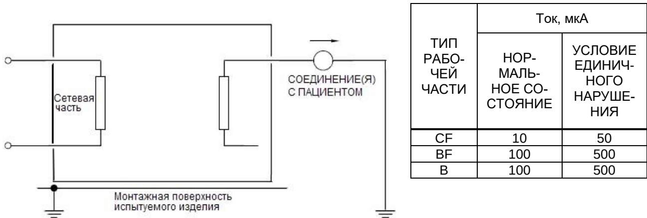
Пример измерительной цепи питания (см. рисунок F.1)
