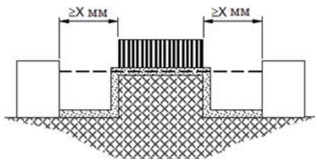
Рисунок 28 – ПУТЬ УТЕЧКИ и ВОЗДУШНЫЙ ЗАЗОР – Пример 7
