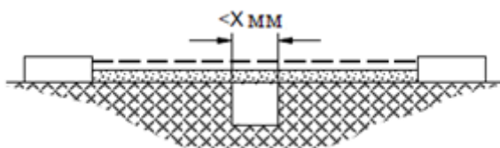
Рисунок 22 – ПУТЬ УТЕЧКИ и ВОЗДУШНЫЙ ЗАЗОР – Пример 1
