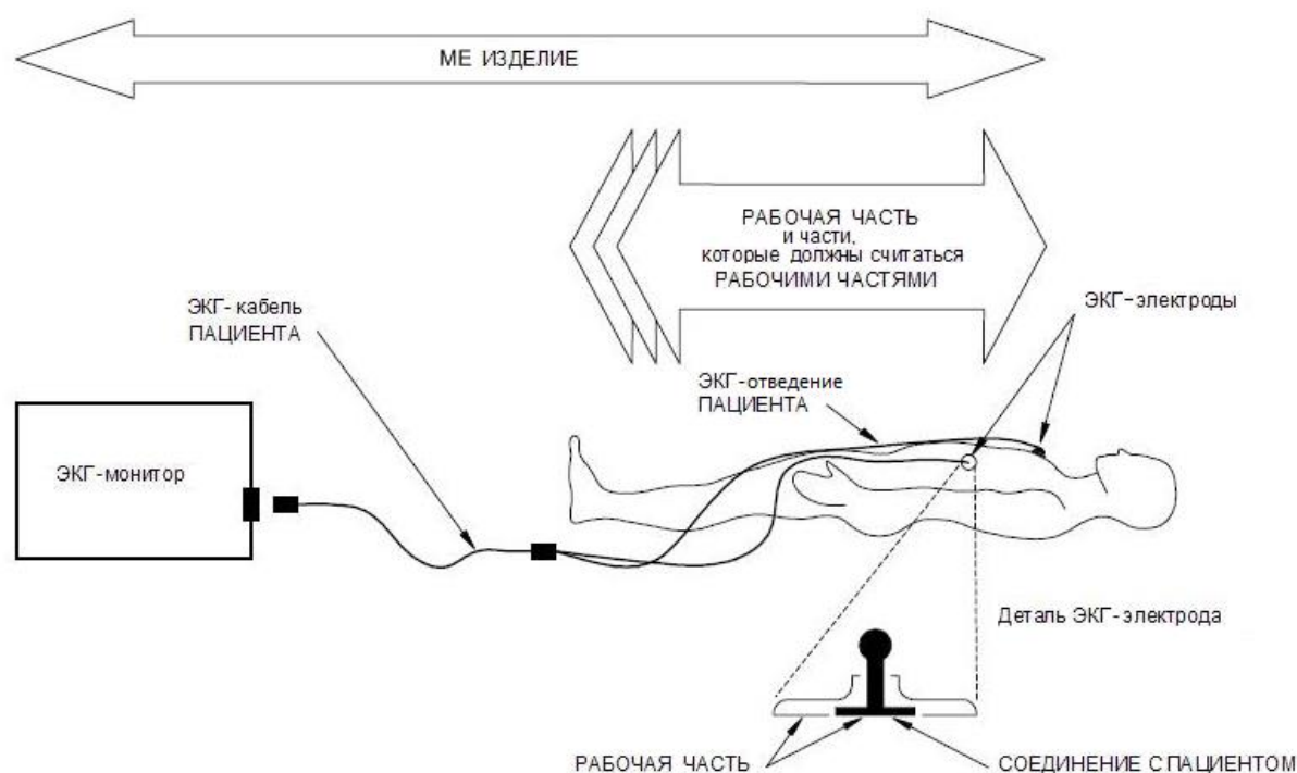
Рисунок А.1 – Идентификация МЕ ИЗДЕЛИЯ, РАБОЧИХ ЧАСТЕЙ и СОЕДИНЕНИЙ С ПАЦИЕНТОМ в ЭКГ-мониторе
