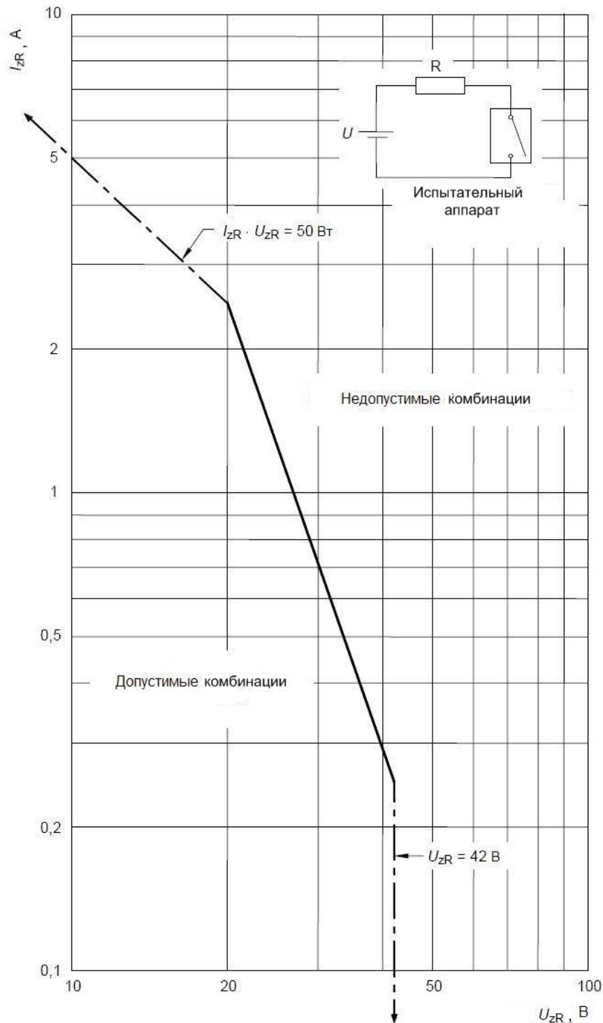
Рисунок G.1 – Зависимость максимально допустимого тока I_{ZR} от максимально допустимого напряжения U_{ZR} , измеренная в чисто активной цепи, находящейся в наиболее воспламеняющейся смеси паров эфира с воздухом
