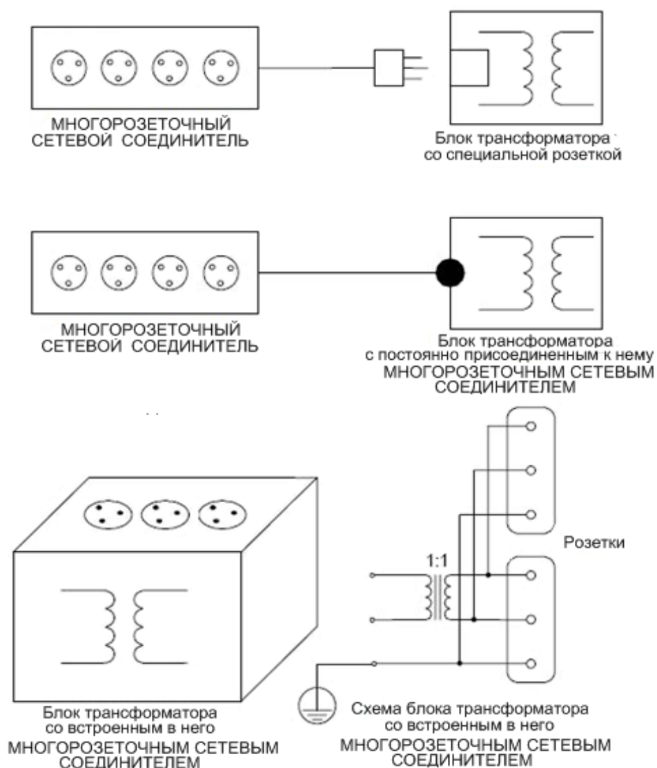
Рисунок I.2 – Примеры применения многорозеточного сетевого соединителя (МСС)
