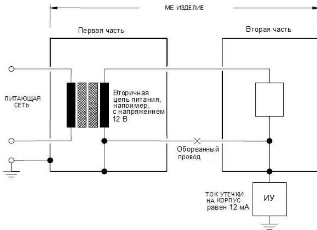
Рисунок А.11 – Обрыв токонесущего провода между частями МЕ ИЗДЕЛИЯ, находящимися в отдельных КОРПУСАХ
