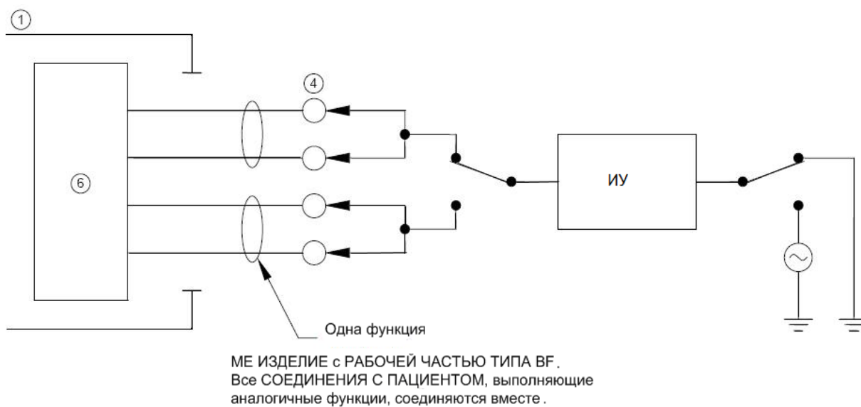
Рисунок Е.1 – Схема присоединения измерительного устройства к МЕ ИЗДЕЛИЮ с РАБОЧЕЙ ЧАСТЬЮ ТИПА В
