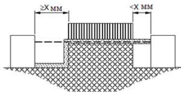
Рисунок 29 – ПУТЬ УТЕЧКИ и ВОЗДУШНЫЙ ЗАЗОР – Пример 8
