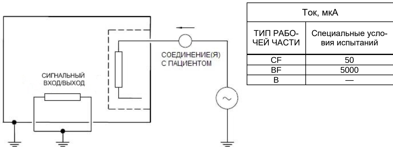
Пример измерительной цепи питания (см. рисунок F.1)
