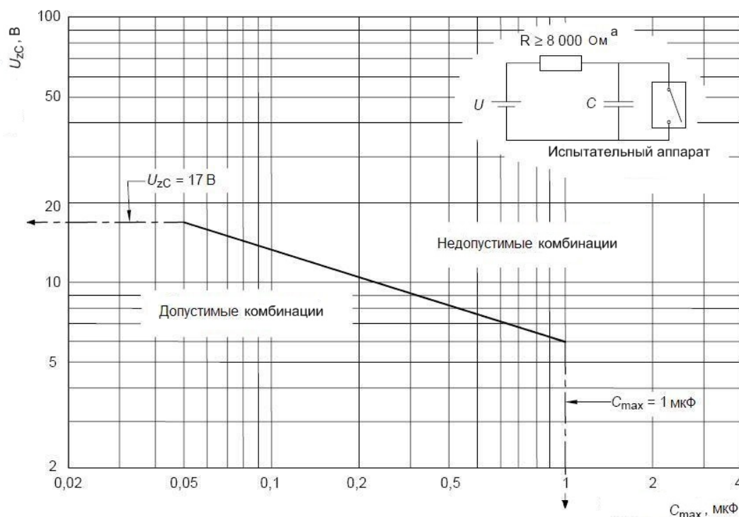
Рисунок G.5 – Зависимость максимально допустимого напряжения U_{ZC} от емкости C_{max} , измеренная в емкостной цепи, находящейся в наиболее воспламеняющейся смеси паров эфира с кислородом
