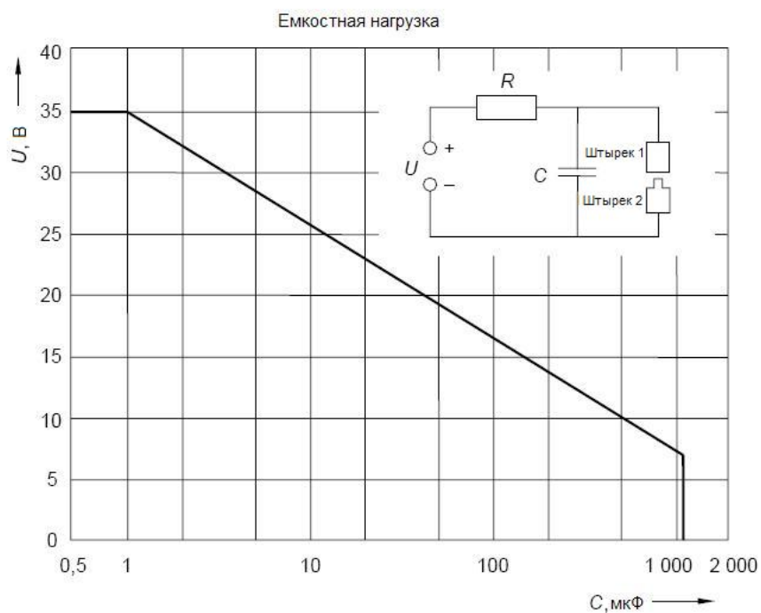
Рисунок 36 – Зависимость максимально допустимого напряжения U от емкости C , измеренная для емкостной цепи в СРЕДЕ С ПОВЫШЕННЫМ СОДЕРЖАНИЕМ КИСЛОРОДА (см. 11.2.2.1)
