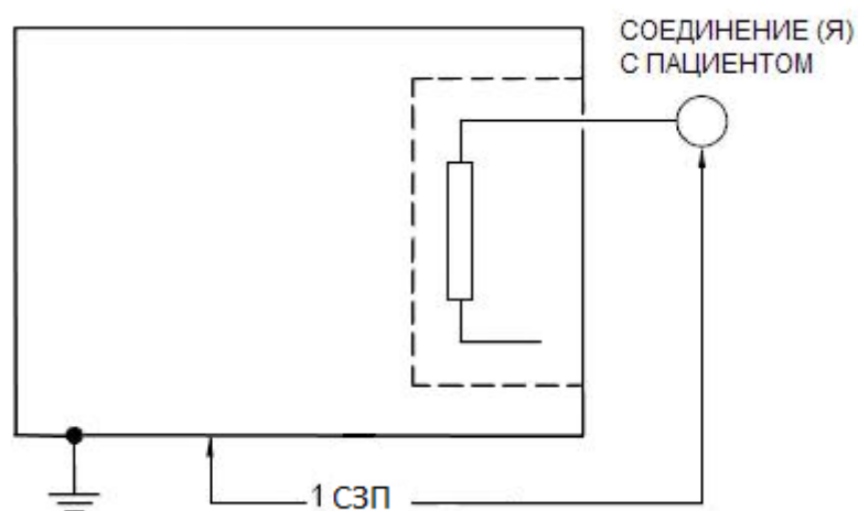
Рисунок J.6 – Пример изоляции 6
