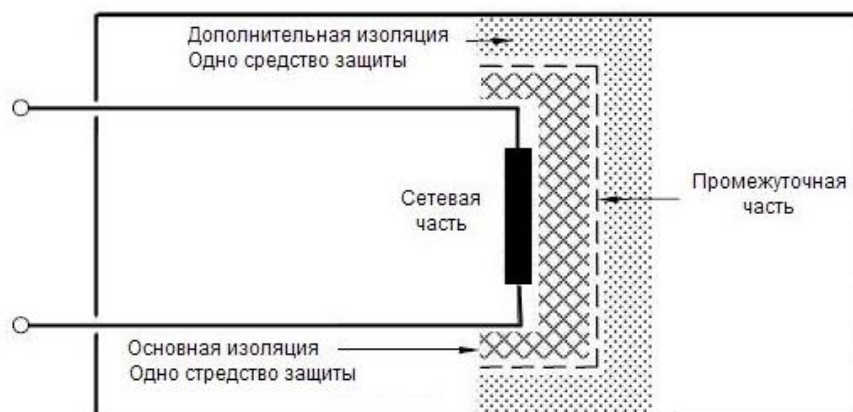
Рисунок J.3 – Пример изоляции 3
