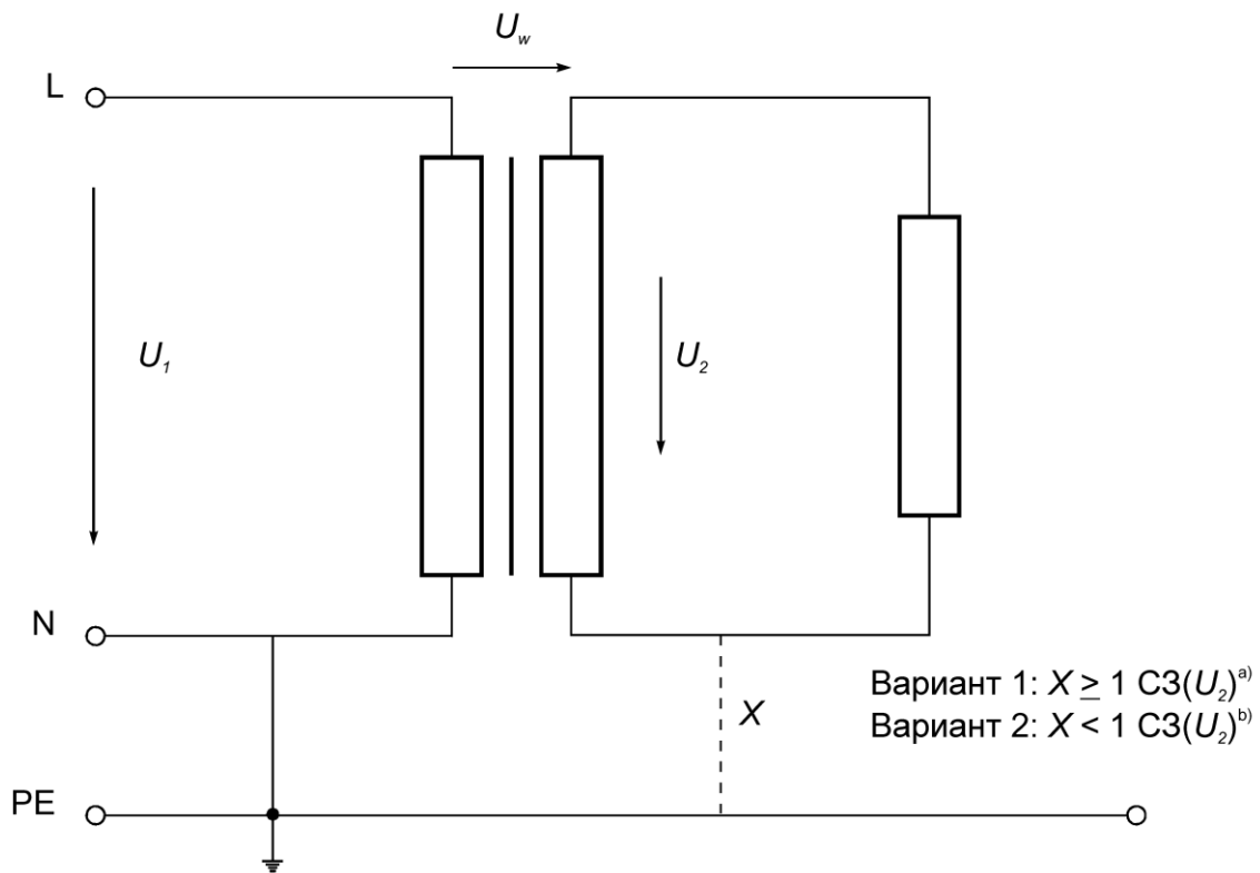
Рисунок 41 — Измерение РАБОЧЕГО НАПРЯЖЕНИЯ
