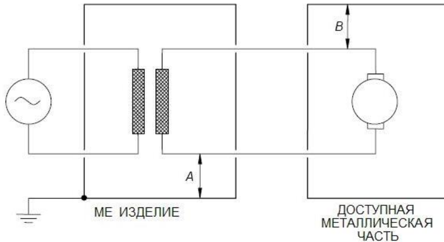
Рисунок А.10 – Пример «плавающей» цепи
