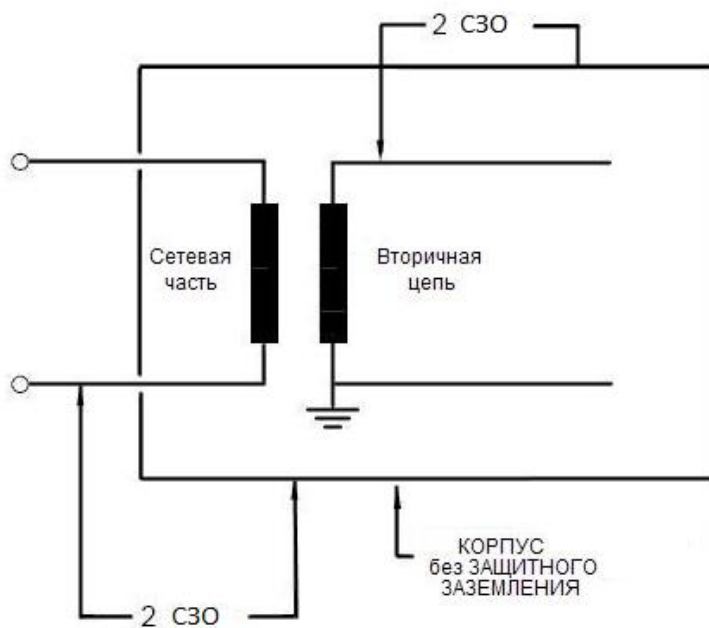
Рисунок J.2 – Пример изоляции 2
