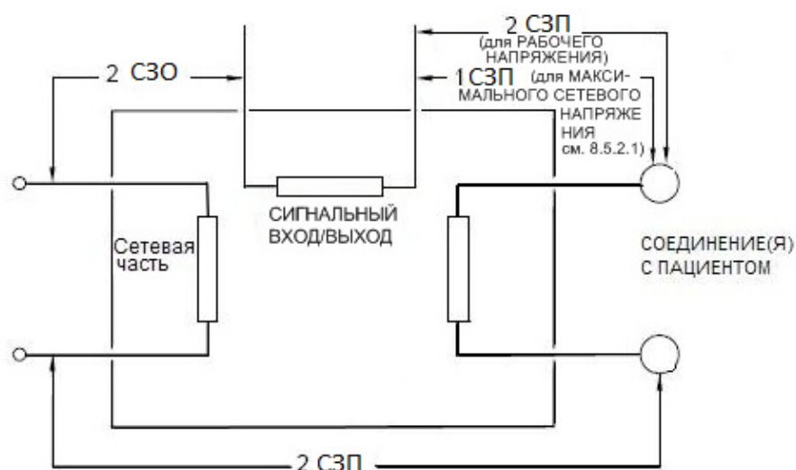
Рисунок J.4 – Пример изоляции 4
