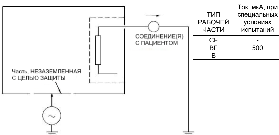
Пример измерительной цепи питания (см. рисунок F.1)
