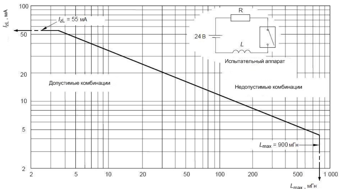
Рисунок G.6 – Зависимость максимально допустимого тока I_{ZL} от индуктивности L_{max} , измеренная в индуктивной цепи, находящейся в наиболее воспламеняющейся смеси паров эфира с кислородом
