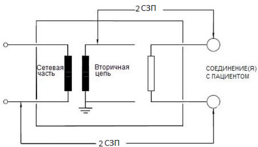
Рисунок J.4 – Пример изоляции 4
