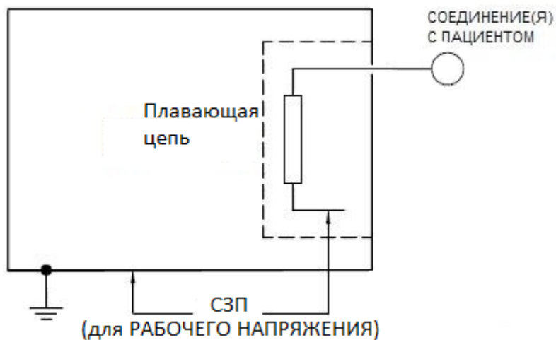
Рисунок J.6 – Пример изоляции 6
