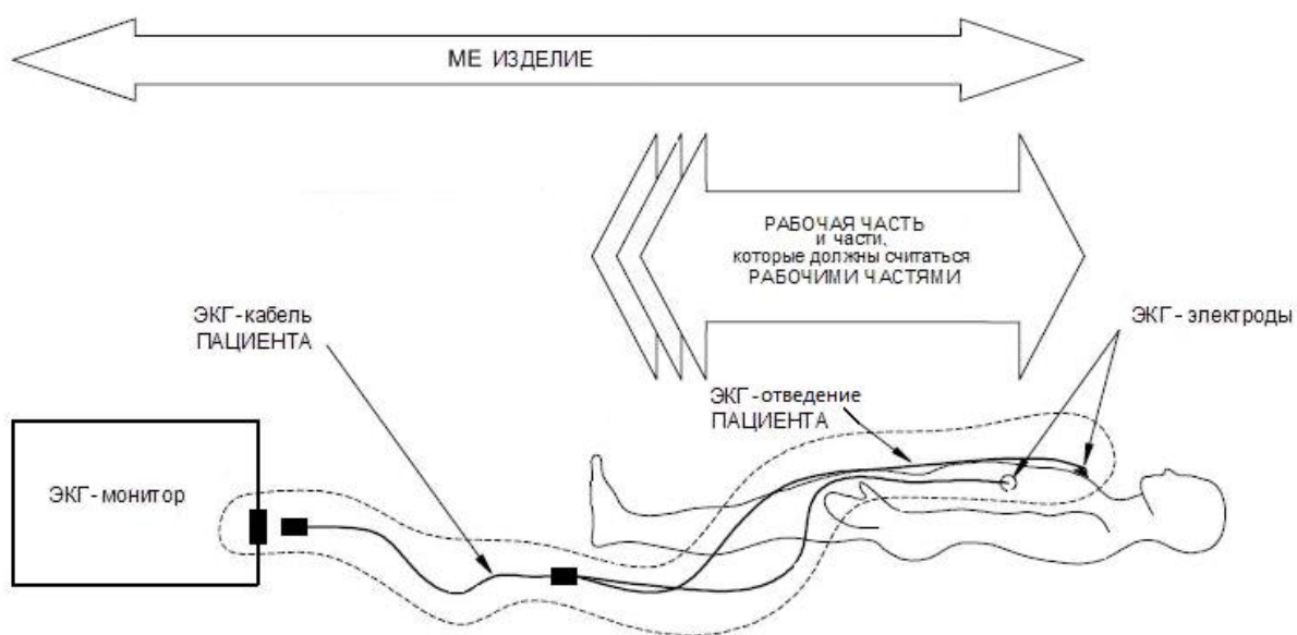
Рисунок А.2 – Пример сочетания изоляции РАБОЧЕЙ ЧАСТИ ТИПА F с изоляцией МЕ ИЗДЕЛИЯ
