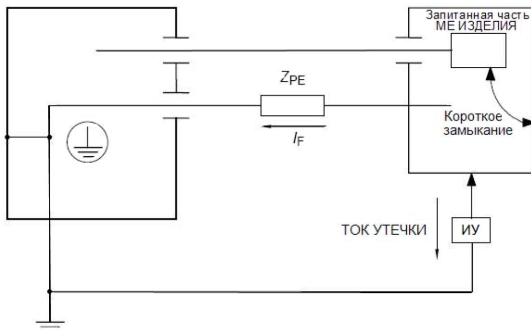
Рисунок А.13 – Допустимый импеданс защитного заземления при ограниченном токе короткого замыкания
