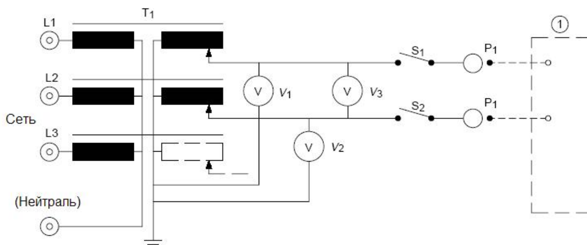
Рисунок F.3 – Измерительная цепь питания многофазного МЕ ИЗДЕЛИЯ, предназначенного для присоединения к многофазной ПИТАЮЩЕЙ СЕТИ (см. 8.7.4.2)
